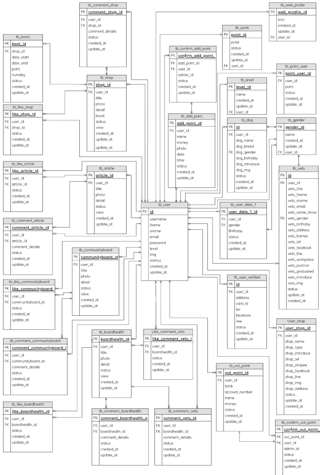
ภาพที่ 3.9 ความสัมพันธ์ของข้อมูล
