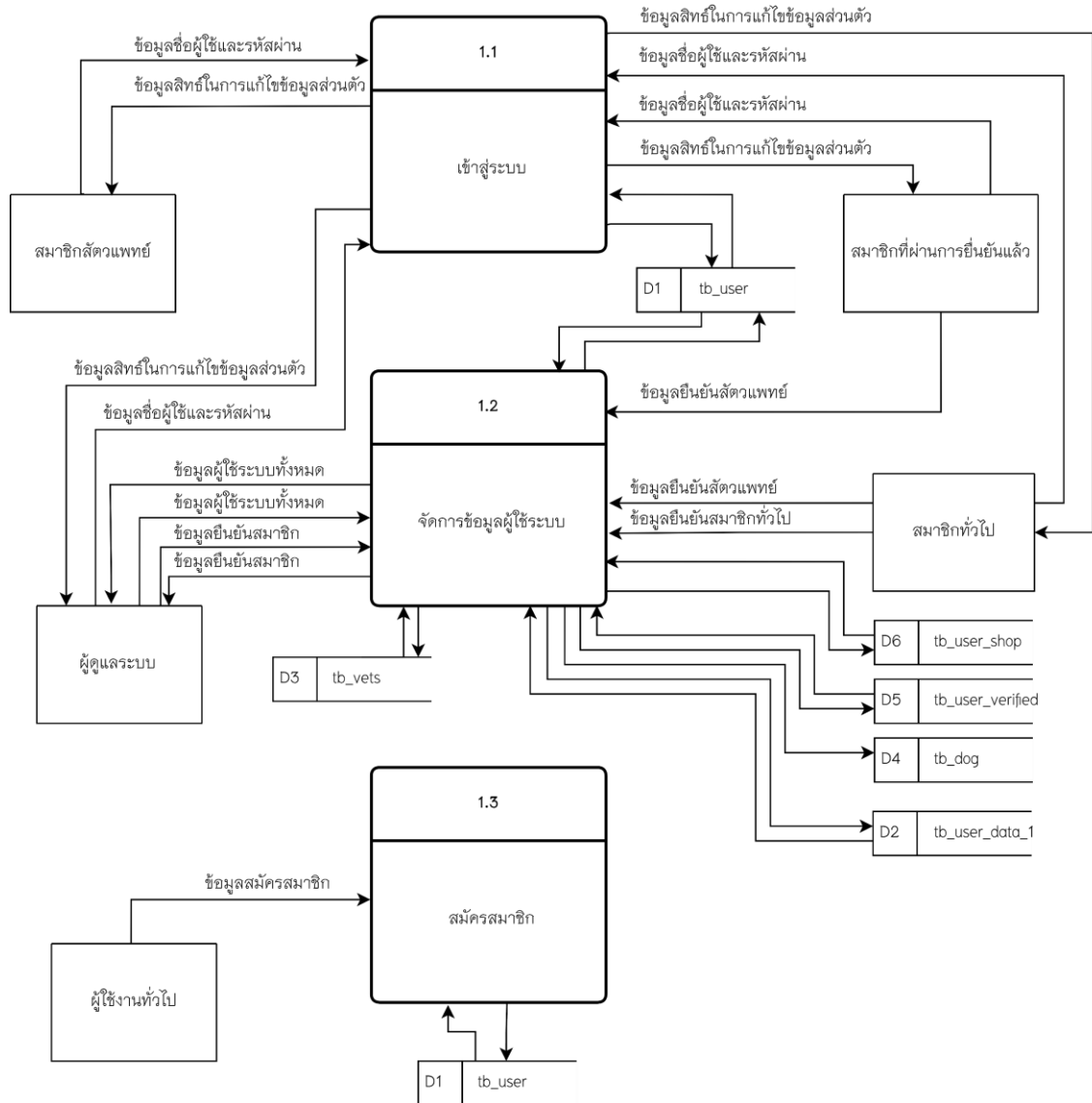
ภาพที่ 3.7 แผนภาพกระแสข้อมูล DFD Level 1 Process 1 จัดการสมัครสมาชิก
