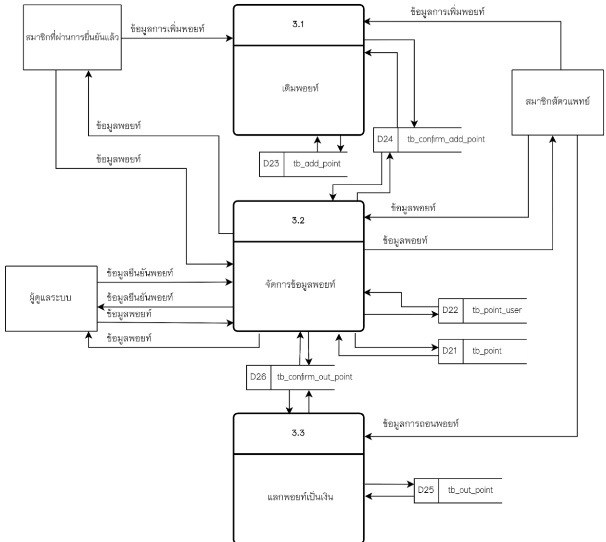
ภาพที่ 3.8 แผนภาพกระแสข้อมูล DFD Level 1 Process 3 จัดการระบบพอยท์และ การแลกพอยท์ของสมาชิกลัทธิแพทย์
